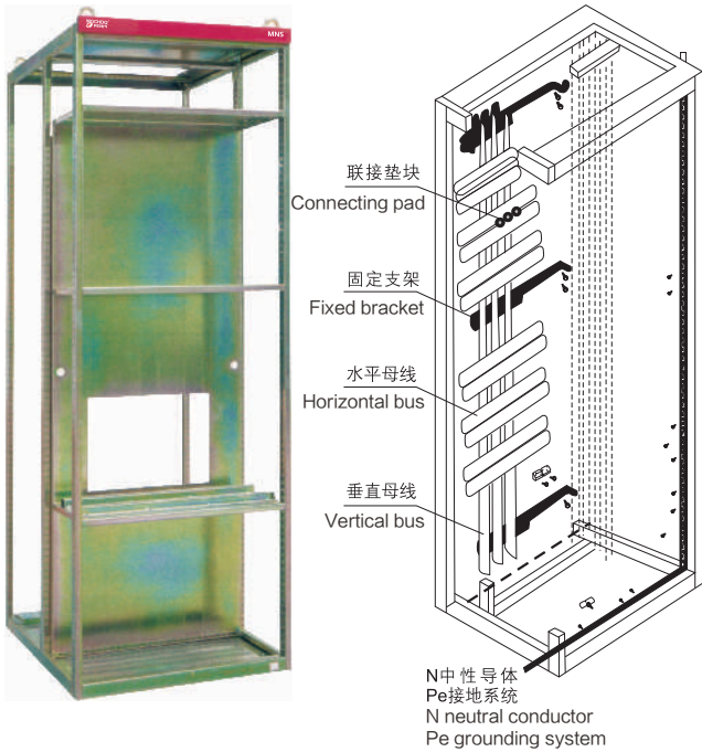
图三、MNS母线系统
