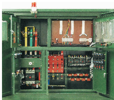
低压室 Low pressure room
