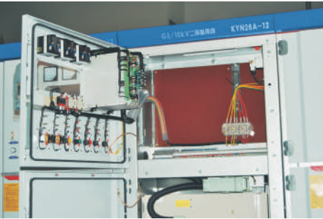
仪表室 Instrument room
