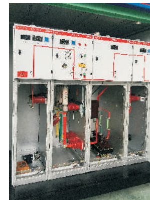
高压室 High pressure chamber
