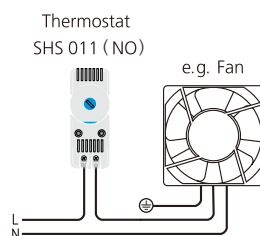
接线示意图 Example of connection
